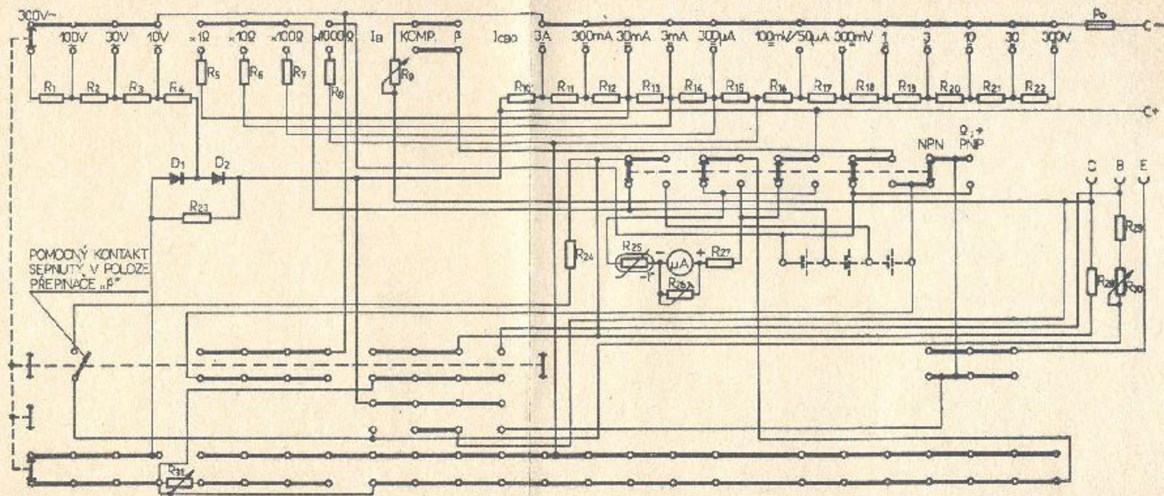
Schéma zapojení ▲
